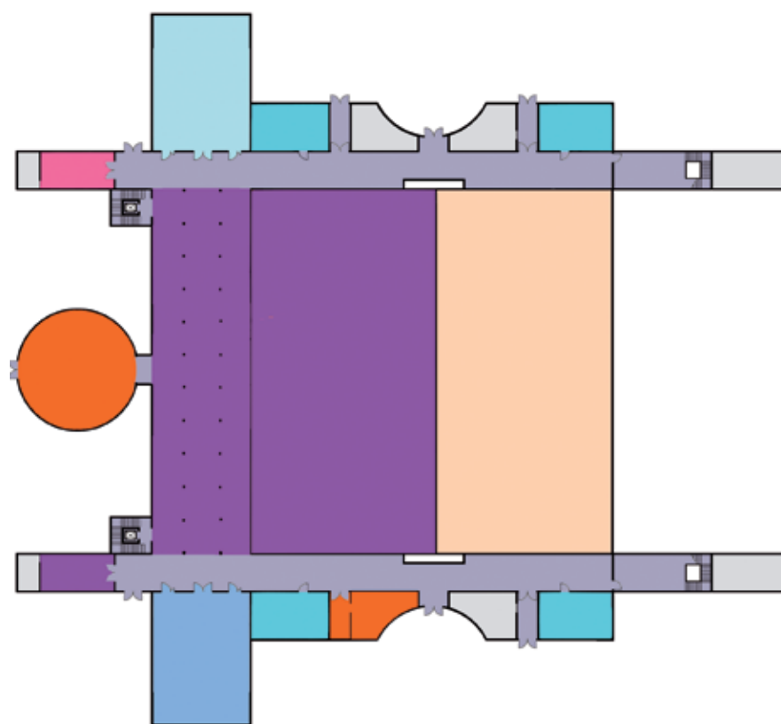
PLANIMETRIA DELLA SEDE CONGRESSUALE PIANO TERRA
